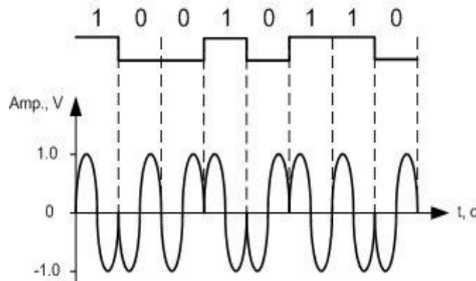
Phase shift keying (PSK)
