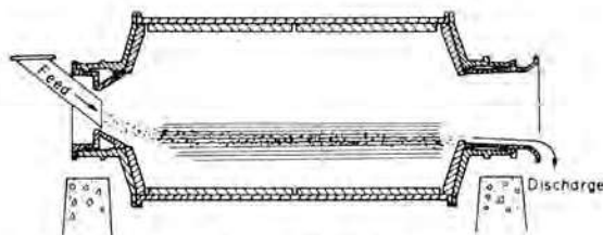
FIG. 7.18. Overflow mill.
