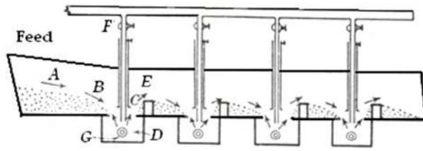
Fig.5.3. Evans Classifier.
