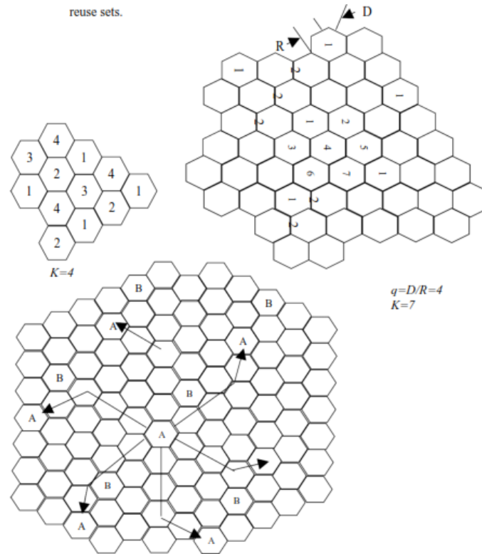
K-CELL REUSE PATTERN
