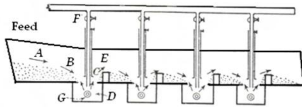
Fig.5.3. Evans Classifier.
